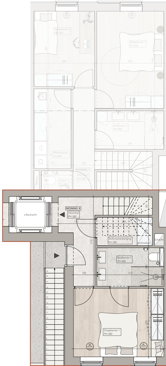
Grondplan LOFTWONING 8
